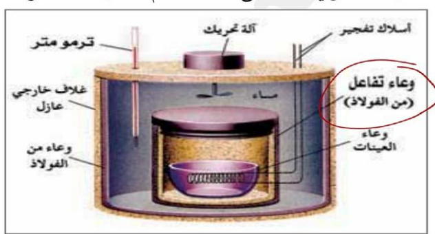
شكل (٧-٢) مسعر القنبلة
