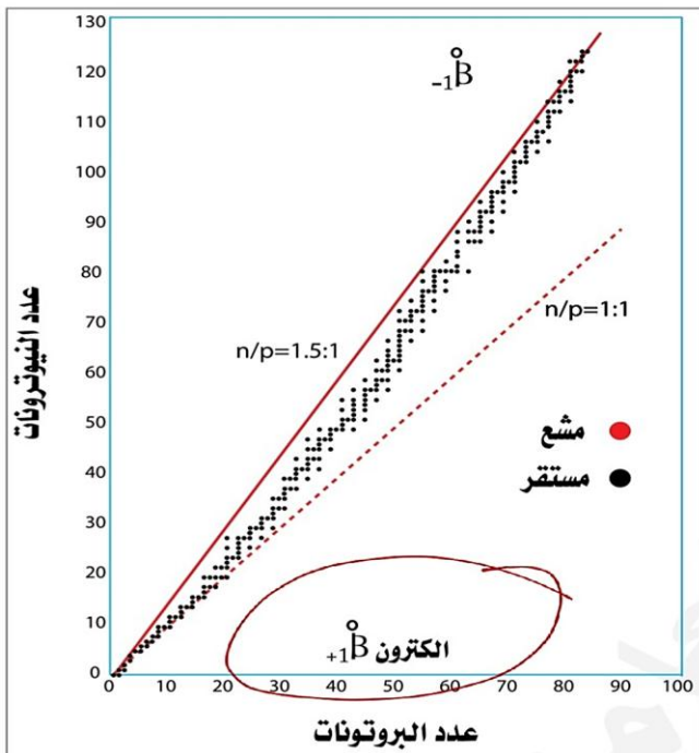
شكل (٣-٤) حزام الاستقرار
