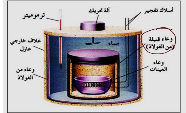
شكل (٧-٢) مسعر القنبلة
